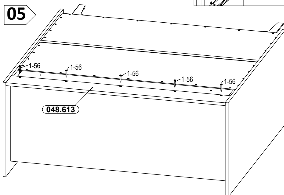
1-56 (Ø4x30)
