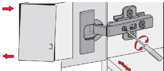
Регулировка дверных петель / Regulacja zawiasów drzwi / Door hinge adjustment
