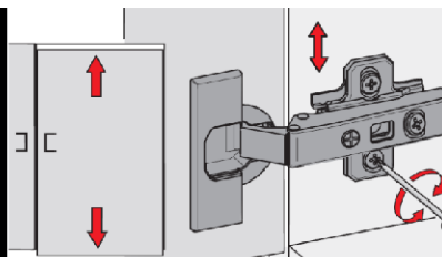
Регулировка дверных петель / Regulacja zawiasów drzwi / Door hinge adjustment
