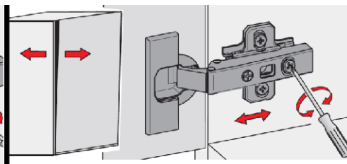
Регулировка дверных петель / Regulacja zawiasów drzwi / Door hinge adjustment
