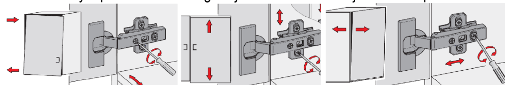
Регулировка петель. Regulacja zawiasów. The adjustment loops.
