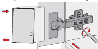
Регулировка петель. Regulacja zawiasów. The adjustment loops.
