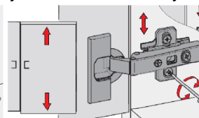
Регулировка петель. Regulacja zawiasów. The adjustment loops.
