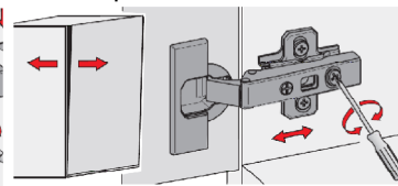
Регулировка петель. Regulacja zawiasów. The adjustment loops.
