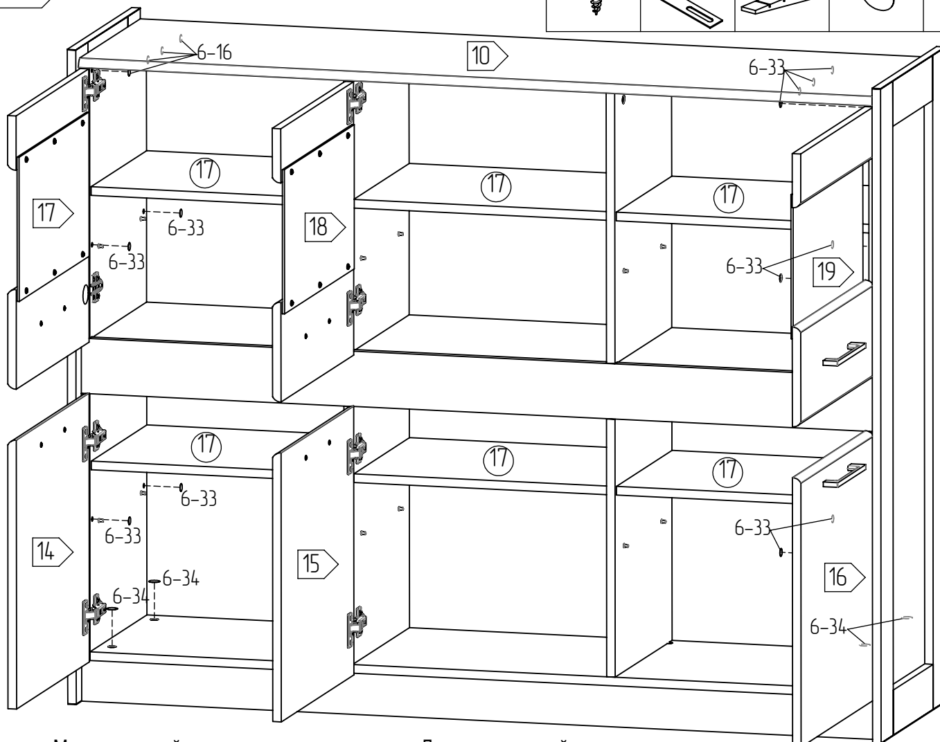
Монтаж дверей на петли
