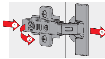
Регулировка петель. Regulacja zawiasów. The adjustment loops.
