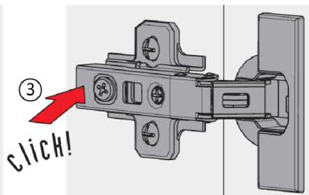
Монтаж дверей на петли Montaż drzwi na zawiasach Installation of doors on hinges
